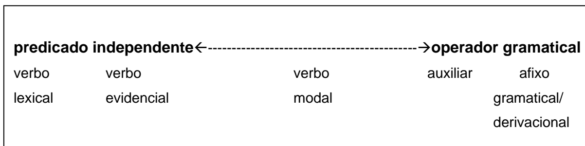
Figura 6 Continuum de gramaticalização (LEHMANN, 1988, p. 204)
